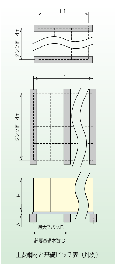
主要鋼材と基礎ピッチ表 (凡例)
