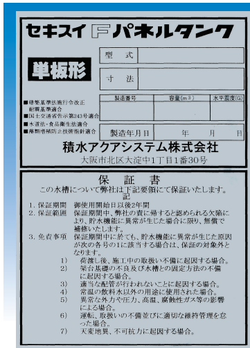
F パネルタンクの銘板および保証書例
