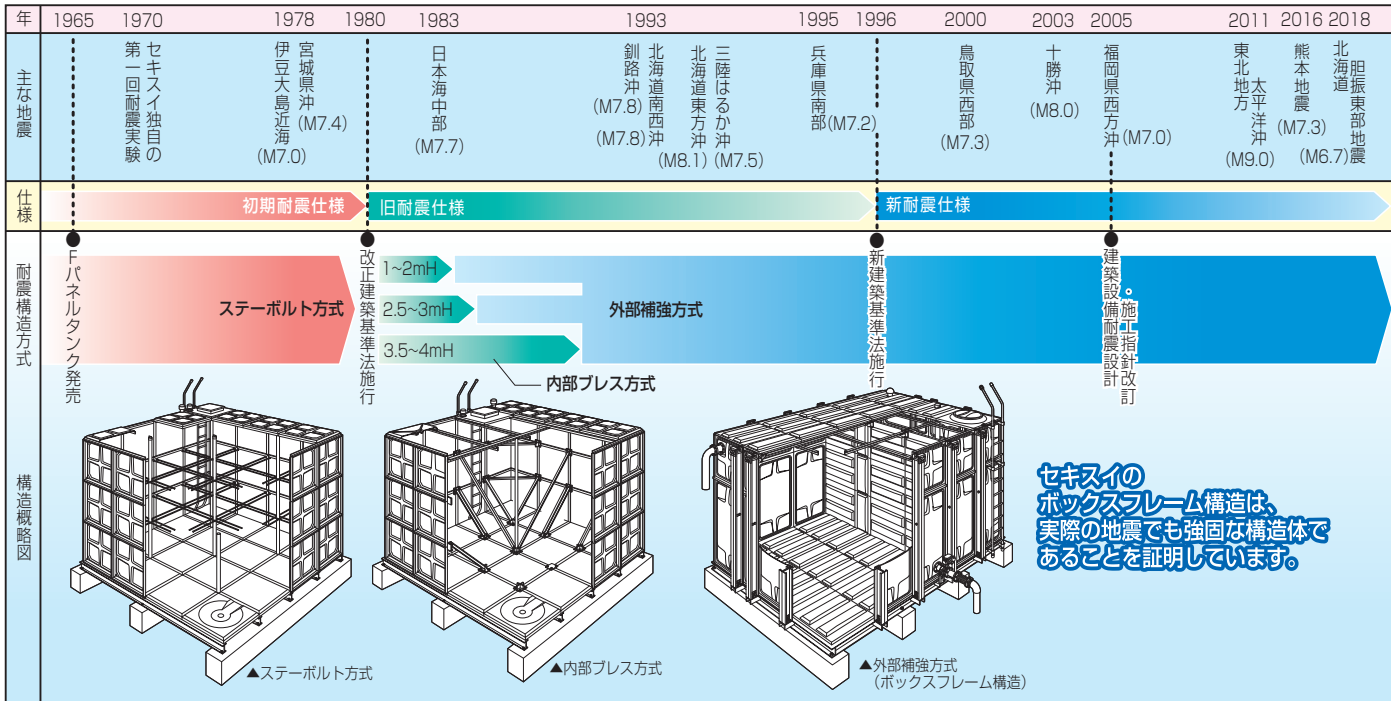
▲外部補強方式 (ボックスフレーム)
