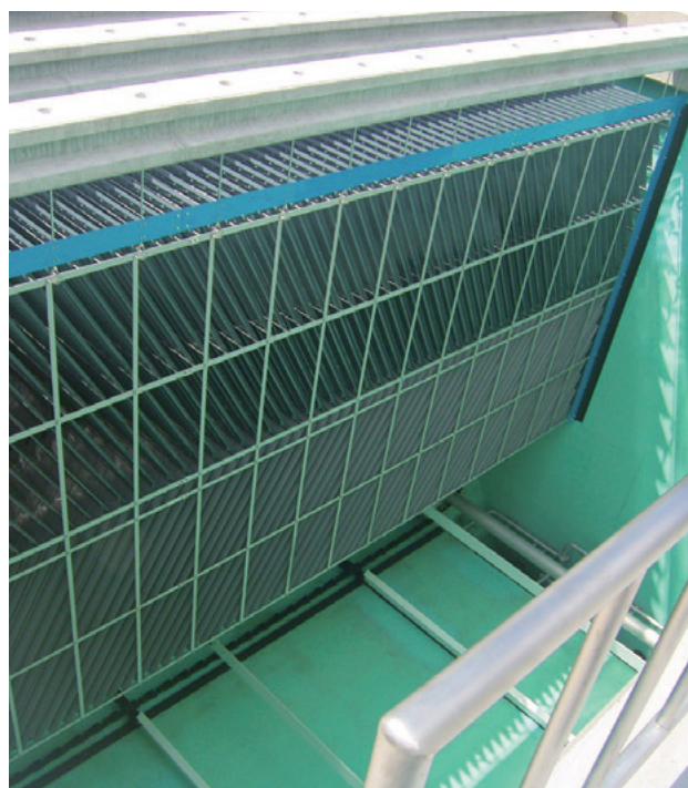
浄水場向け傾斜板沈降装置(横向流式・長尺仕様)
