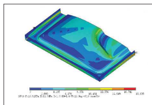
▲1×1mパネル FEM解析
