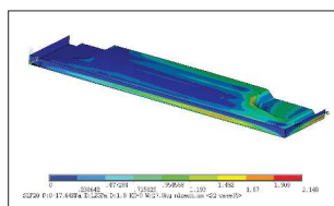
▲1×2mパネル FEM解析
